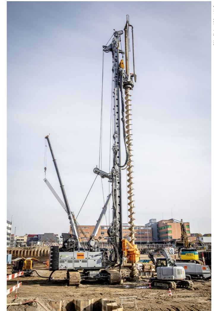
Ein Kran (Hintergrund) transportiert den 25 Meter langen Armierungskorb zum Bohrloch. Der Sennebogen 653 E kann bis 9,2 Tonnen Gewicht heben.
