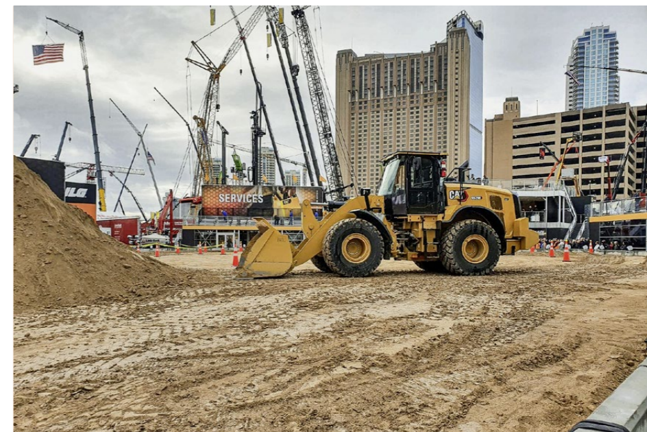
Erste Finalprüfung: Bruno Grossen beim Beladen eines Muldenkippers mit dem Cat Radlader 962M.
